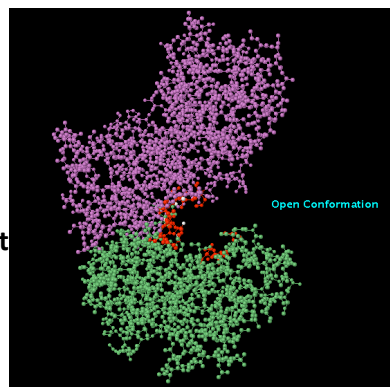
conformation ouverte
