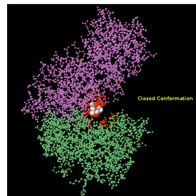
conformation fermée
